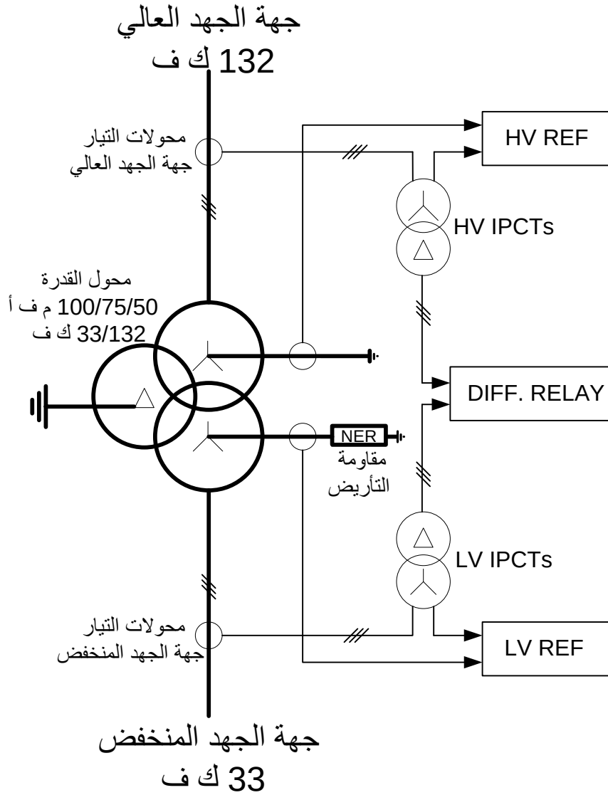
شكل رقم (59): توصيل جهاز الحماية المقيدة ضد التسرب الأرضي من نفس محولات التيار المستخدمة في جهاز الحماية التفاضلية لمحول القدرة
