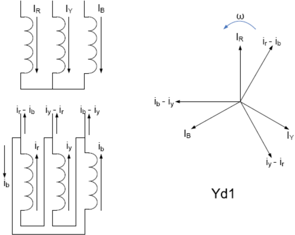
شكل رقم (18): توصيلة محول قدرة ثلاثي الأوجه بطريقة Yd1
